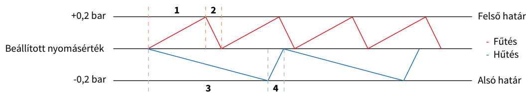
* Fűtési rendszer grafikonja.
